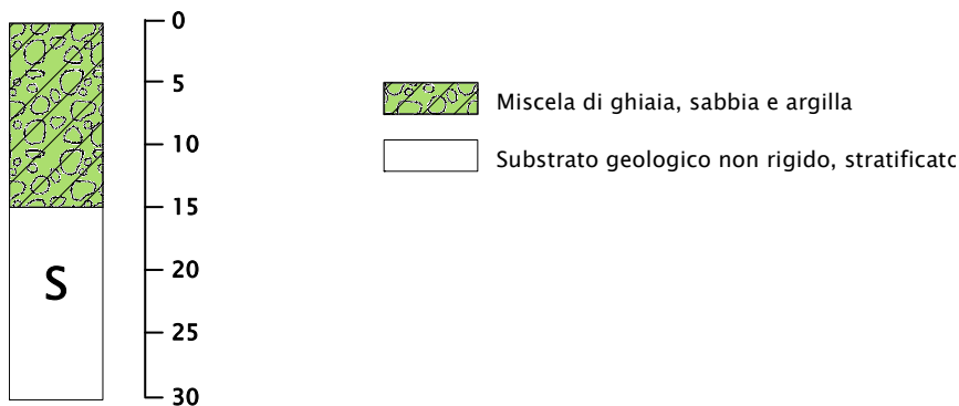
Figura 36 – Successione stratigrafica cod. 2002.
