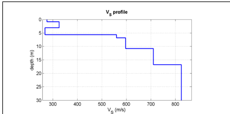
Figura 49 – Profilo tipo di Vs delle aree individuate come zone stabili (1041). Substrato a 5.7m, MASW 036025L58.
