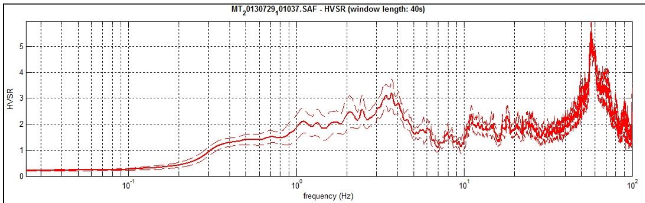
Figura 32 - Curva H/V rappresentativa dei valori di frequenza compresi tra 2-8 Hz. Picco a 3.7 Hz, HVSR 036025P287.
