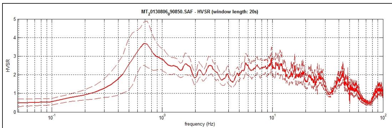
Figura 31 – Curva H/V rappresentativa dei valori di frequenza minori di 1 Hz. Picco a 0.8 Hz, HVSR 036025P311.
