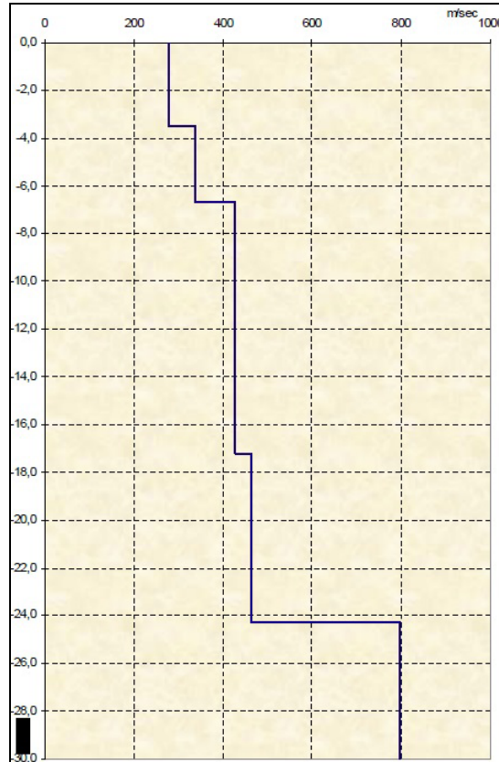
Figura 48 – Profilo tipo di V_s delle aree con depositi (Zona 2001) o frane. Substrato a 24.4m, MASW 036025L23.
