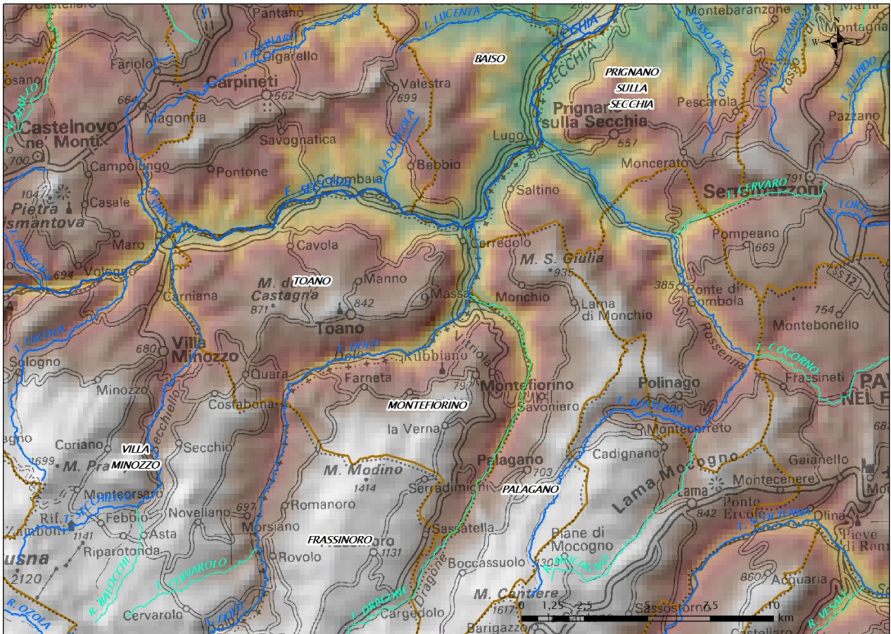
Figura 2 – Inquadramento geografico-fisico del territorio comunale di Montefiorino. Il DEM (modello digitale delle quote) mostra le differenti fasce altimetriche: da quelle con valori relativamente più alti, in grigio chiaro, a quelle con i valori relativamente più bassi, in verde e azzurro.
