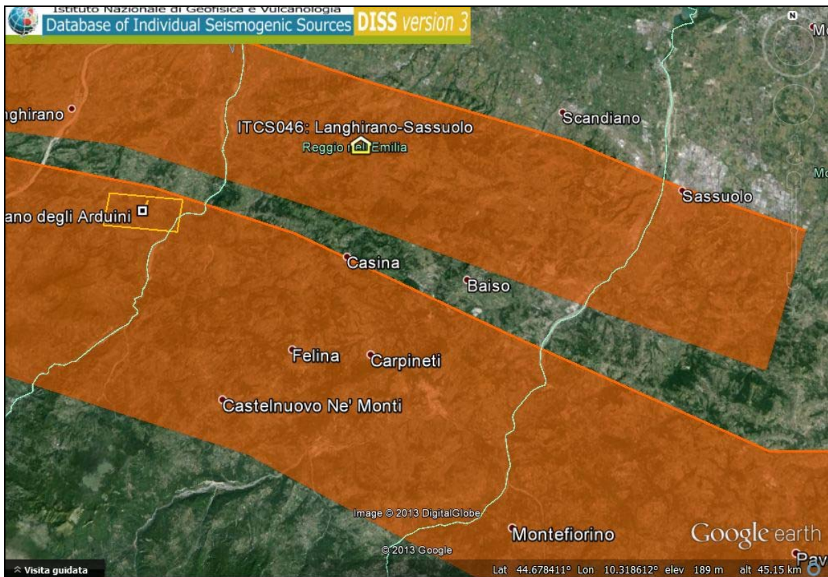
Figura 9 – Estratto dal database of Individual Seismogenic Sources (DISS) dell'INGV: tratto della Sorgente Sismogenetica Composita (ITCS) 046 “Langhirano–Sassuolo”.
