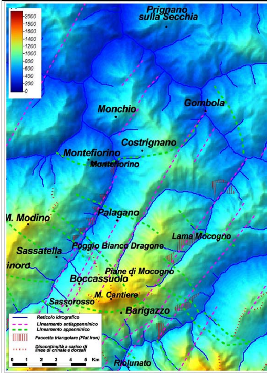
Figura 18 – Rappresentazione della topografia dell'area compresa tra la Val Dragone e la Valle dello Scoltenna tramite modello digitale del terreno (fonte dati: DEM SRTM, sito web NASA). Da: “Indagine geologico – ambientale”, a cura dello Studio Geologico Ambientale “Arkigeo” del Dott. Geol. Giorgio Gasparini, per il redigendo Piano Strutturale Comunale dell’Unione di Comuni Montani “Valli Dolo, Dragone e Secchia” (Montefiorino, Palagano e Prignano sulla Secchia).
