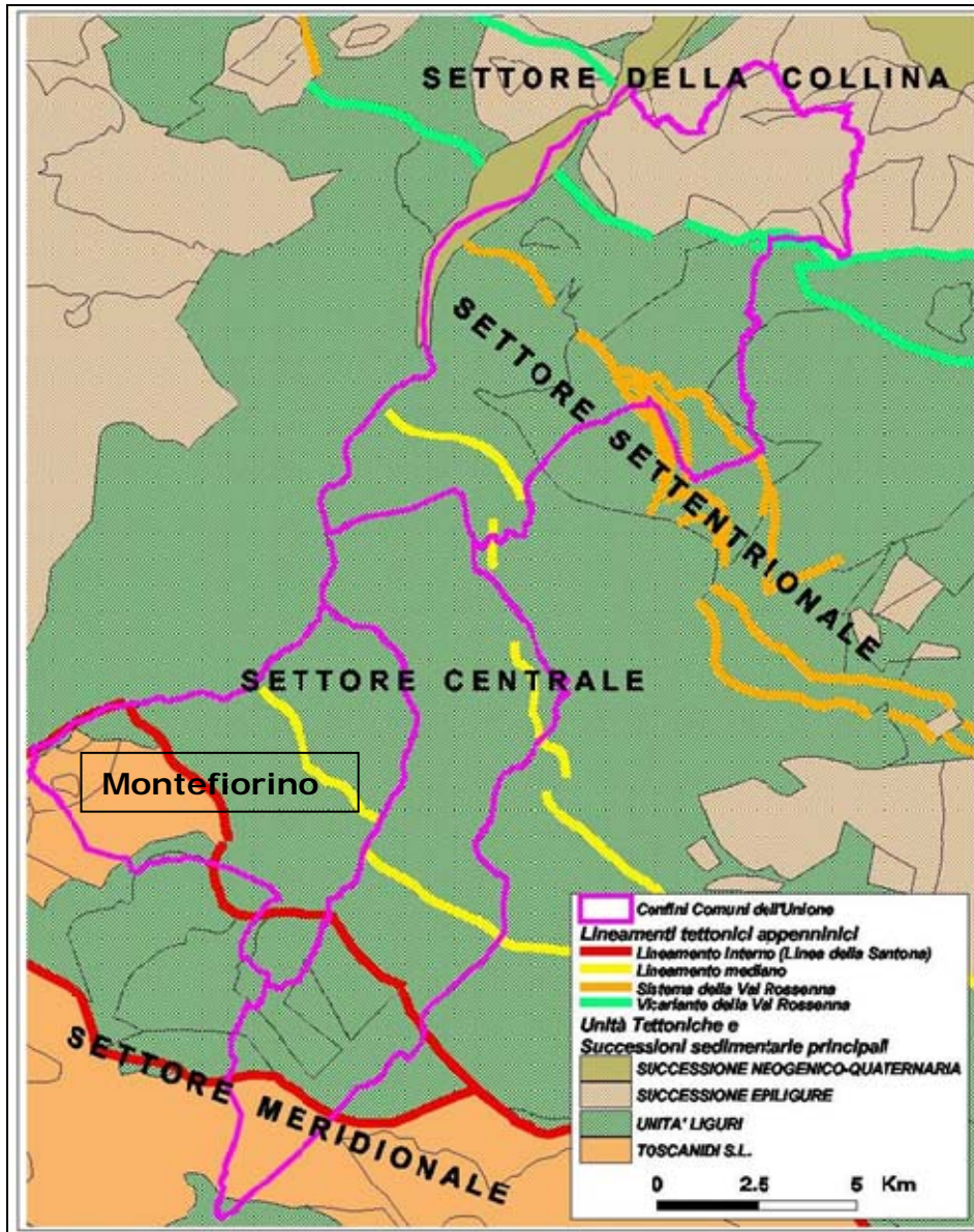
Figura 16 – Schema tettonico del settore centro occidentale dell'Appennino Modenese (fonte: "Indagine geologico - ambientale", a cura dello Studio Geologico Ambientale "Arkigeo" del Dott. Geol. Giorgio Gasparini, per il redigendo Piano Strutturale Comunale dell'Unione di Comuni Montani "Valli Dolo, Dragone e Secchia" (Montefiorino, Palagano e Prignano sulla Secchia).
