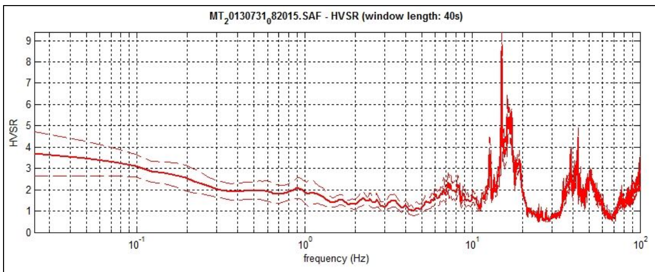
Figura 33 - Curva H/V rappresentativa dei valori di frequenza maggiori di 8 Hz. Picco a 15 Hz, HVSR 036025P314.
