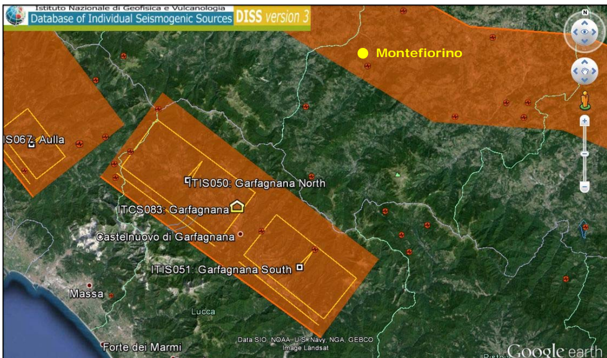
Figura 8 – Estratto dal database of Individual Seismogenic Sources (DISS) dell'INGV: Sorgente Sismogenetica Composita (ITCS) 083 “Garfagnana” e Sorgenti Sismogenetiche Individuali (ITIS) 050 “Garfagnana Nord” e 051 “Garfagnana Sud”.
