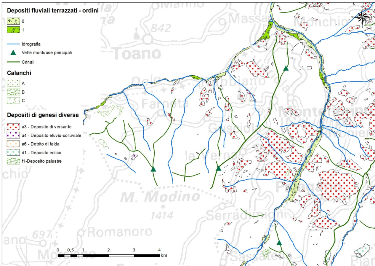
Figura 22 – Distribuzione dei depositi alluvionali terrazzati (solo ordini minori), dei depositi di genesi diversa e dei calanchi nel territorio comunale di Montefiorino. Tematismi vettoriali estratti dalla Carta Idro-geomorfologica del redigendo PSC dell’Unione dei Comuni delle Valli Dolo–Dragone–Secchia.
