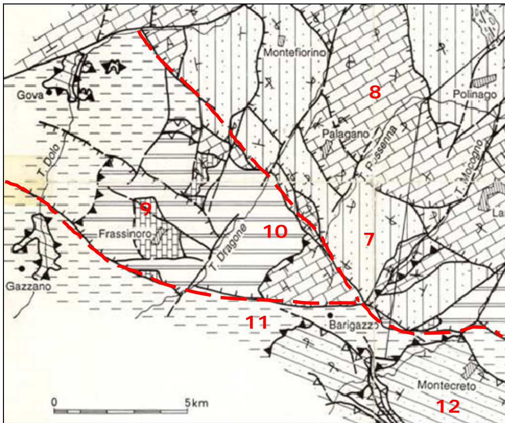
Figura 17 – Carta Geologico-strutturale schematica – estratto da (Bettelli e Panini, 1992). Legenda: 7) Formazione di Monghidoro; 8) Formazione di Monte Venere, 9) Flysch di Monte Caio, 10) Complesso di base I: Arenarie di P.gio Castellina (Arenarie di Frassinoro), Argilliti di P.gio Mezzature, argilliti variegata, torbiditi arenaceo-pelitiche, Argille a palombini; 11) Unità tettonica Sestola-Vidiciatico (Unità Ventasso); 12) Arenarie di Monte Cervarola. Elementi lineari: linea continua-faglia subverticale o trascorrente; linea con triangoli vuoti-Faglia inversa; linea con triangoli pieni-sovrascorrimento; linea con linee tratteggiate-faglia normale. La linea rossa tratteggiata individua il Lineamento Interno (o Linea della Santona) che a ovest di Barigazzo si suddivide in due diramazioni.
