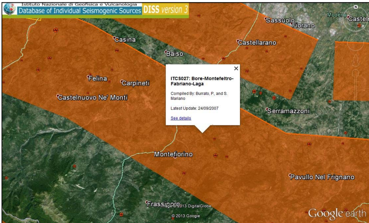
Figura 7 – Estratto dal database of Individual Seismogenic Sources (DISS) dell'INGV: tratto della Sorgente Sismogenetica Composita (ITCS) 027 “Bore–Montefeltro–Fabriano–Laga”.
