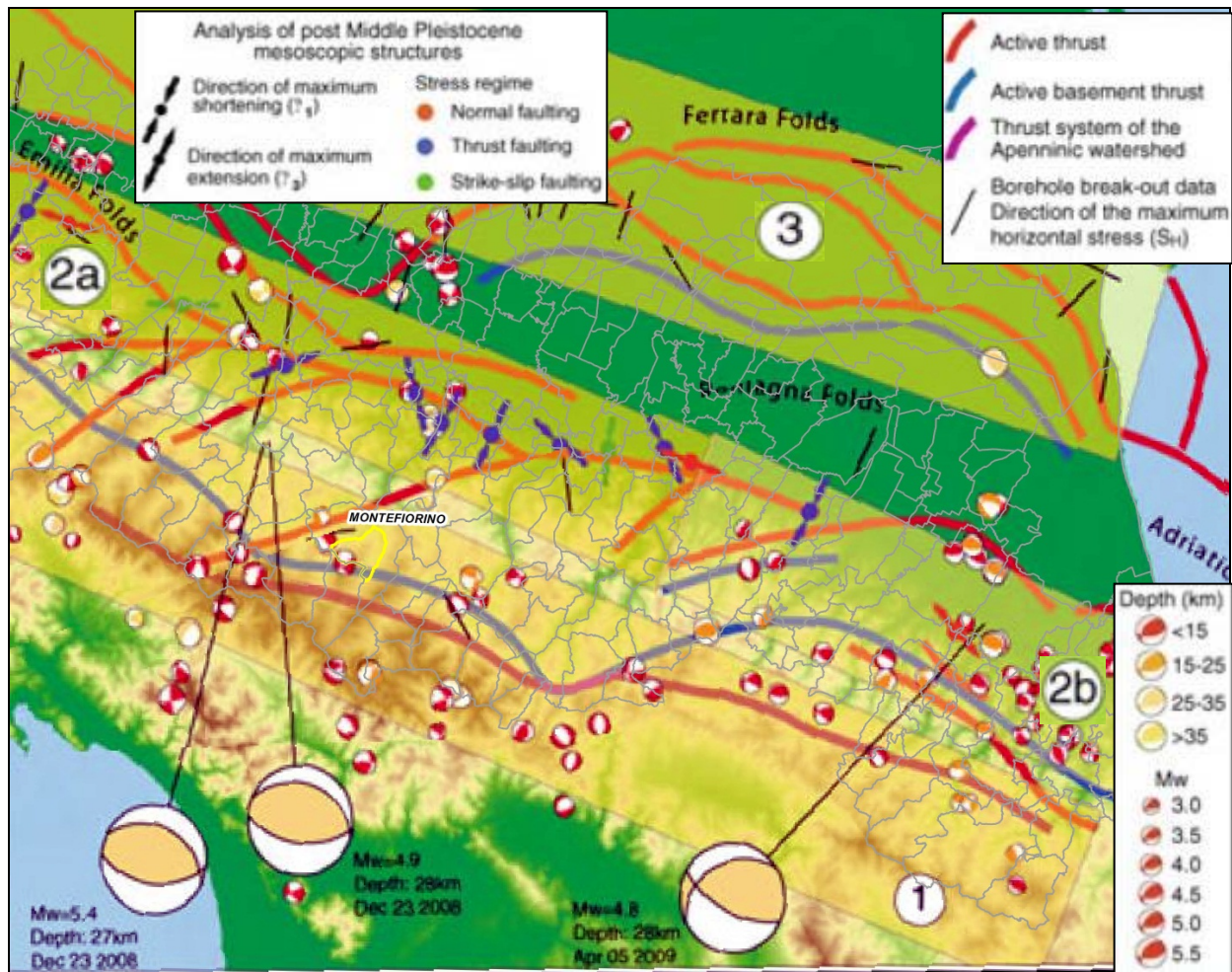
Figura 3 – Sintesi delle strutture recenti e attive del settore esterno degli Appennini settentrionali, con sovrapposte le soluzioni dei meccanismi focali (Boccaletti et al., 2004), i campi tensionali da analisi mesoscopiche (Ghiselli e Martelli, 1997) e i dati di breakout da pozzo (Mariucci e Muller, 2003). Tre meccanismi focali in dettaglio relativi agli eventi principali di sequenze sismiche che hanno interessato gli Appennini il 23 dicembre 2008 ed il 5 aprile 2009 (da dati INGV). I numeri nei cerchi indicano i principali sistemi di faglie: (1) Catena appenninica; (2a) Margine Appennini–Pianura (settore nord–occidentale); (2b) Margine Appennini–Pianura (settore sud–orientale); (3) Pieghe Emiliane e Ferraresi sepolte. (Fonte: Boccaletti et al., 2011). Il poligono con contorno giallo individua in carta il territorio comunale di Montefiorino.
