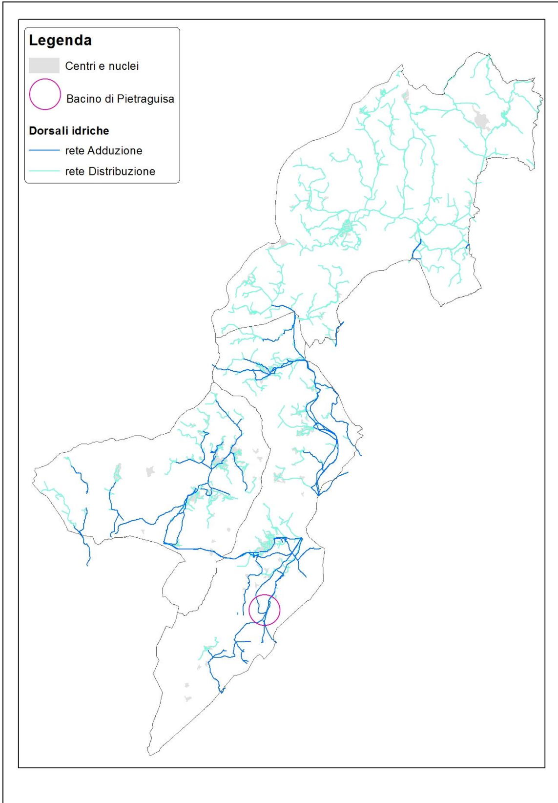
Dorsali di distribuzione dell'acqua nel territorio dei tre comuni Fonte: Relazione di quadro conoscitivo Sistema insediativo. Elaborazione propria su valutazioni e indicazioni di HERA 2014
