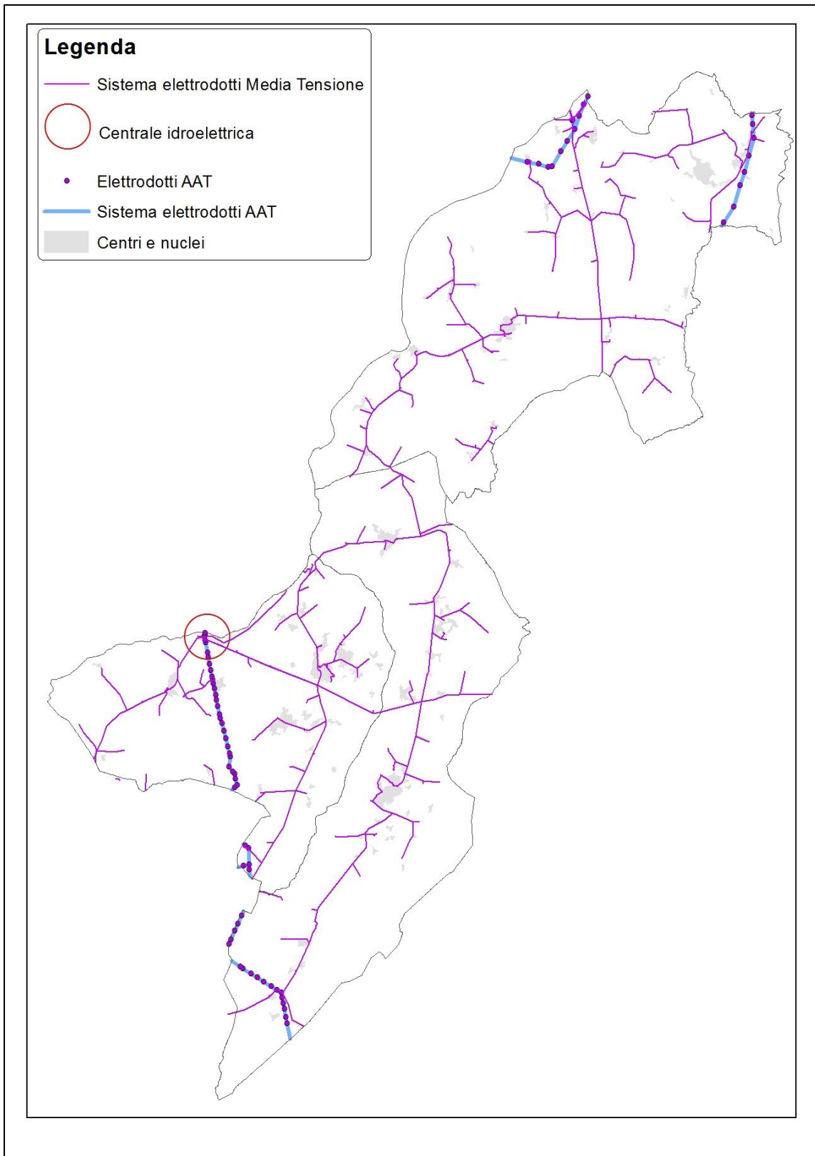
Rete di distribuzione dell'energia elettrica ad alta e media tensione Fonte: Relazione di quadro conoscitivo Sistema insediativo. Elaborazione propria da quadro conoscitivo del PTCP
